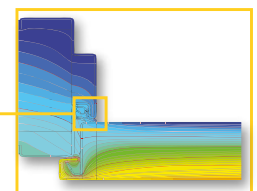
standardowa ościeżnica
