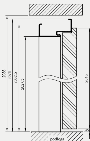
Przekrój poprzeczny alternatywny sposób montażu
