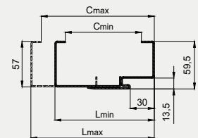
Profil ościeżnicy stalowej regulowanej z kątownikiem domykającym T57
