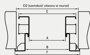
Przekrój poprzeczny przy montażu na zaprawę murarską
