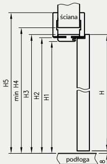
Przekrój pionowy OR
