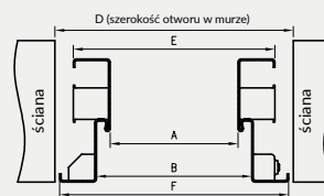
Przekrój poprzeczny przy montażu na wełnę mineralną
