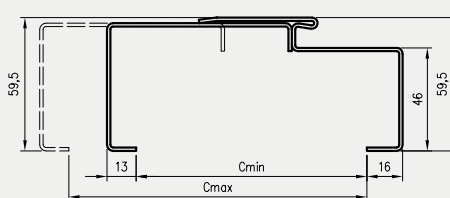
profil ościeżnicy
