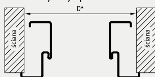
Przekrój poprzeczny alternatywny sposób montażu
