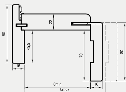
Profil ościeżnicy
