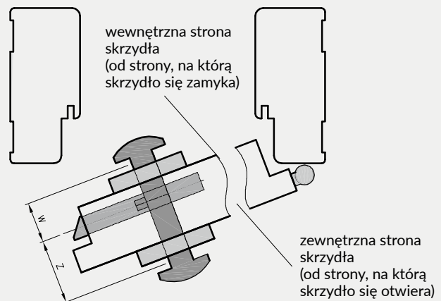
Rys. Dobór wymiaru wkładki z gałką
