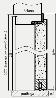
Przekrój pionowy przy montażu na zaprawę murarską
