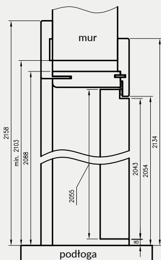
Przekrój pionowy ORO
