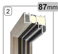
Ościeżnica aluminiowa ALU/90 trzykomorowa z podwójnym uszczelnieniem z przegrodą PCW wypełniona pianą
