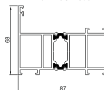
Profil naświetla
