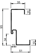
Ościeznica stalowa 10/54, 10/54 AKU
