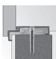
ościeżnica Kątowa DUŻA montaż na dyble
