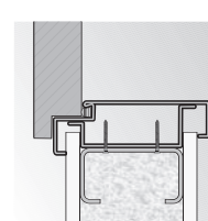
ościeżnica Kątowa DUŻA montaż na ścianie kartonowo-gipsowej
