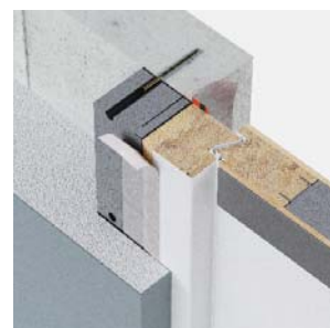
system pasywny (stojak)
