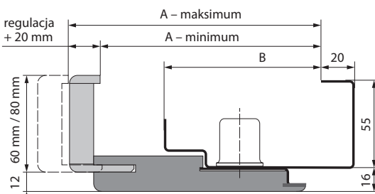
przekrój ościeżnicy PROJEKT Premium
