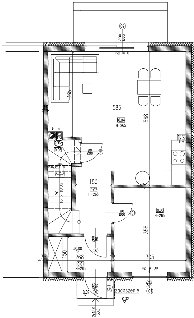
Budynek 6 - Kondygnacja 0
